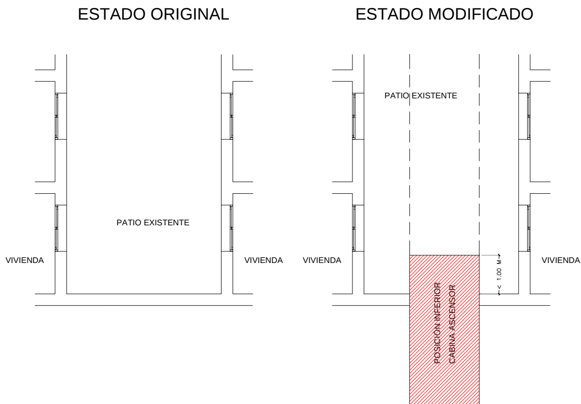
Grafico 2: Instalación de Ascensor en patio interior con viviendas en Planta Baja. Caso Genérico.
